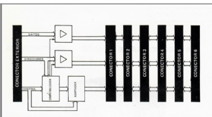
Diagrama de bloques del CR-401
